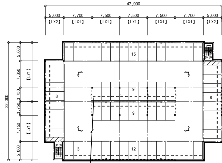
2階 平面図
